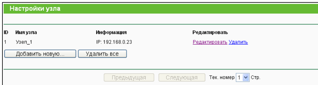
Рис. 4-53 Настройки узла
